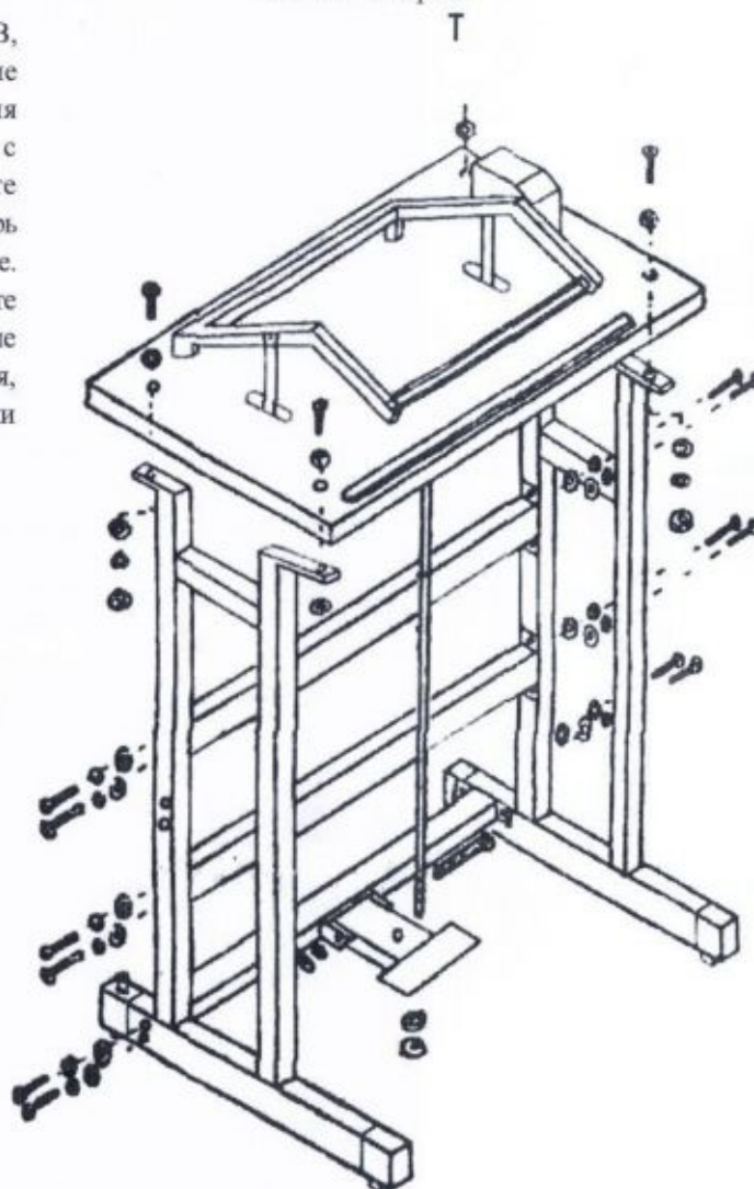
Схема сборки
