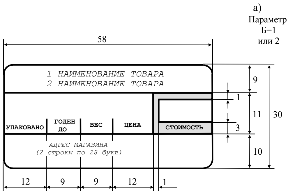
Рис.4. ВИД ЭТИКЕТОК С ПАРАМЕТРОМ А=1 ( размеры в мм )
