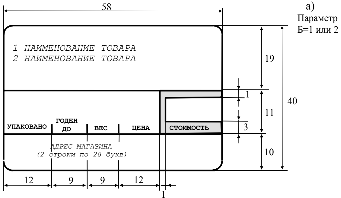
Рис.6. ВИД ЭТИКЕТОК С ПАРАМЕТРОМ А=3 (размеры в мм)
